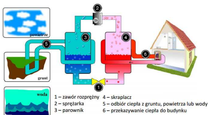
Rysunek 14 Zasada działania pompy ciepła 171
