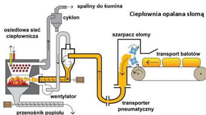
Rysunek 17 Schemat kotłowni na słomę 179
