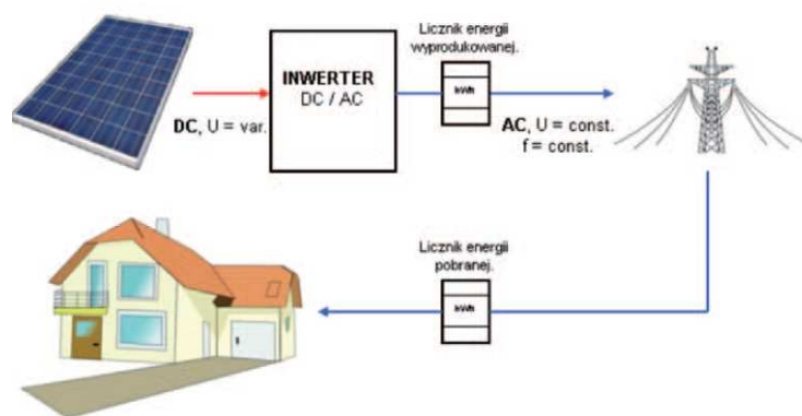
Rysunek 22 Schemat instalacji ON-GRID 188 (oznaczenia: DC- prąd stały, AC-prąd przemienny, U- napięcie, f-częstotliwość, var.-zmienne, const.- stałe)
