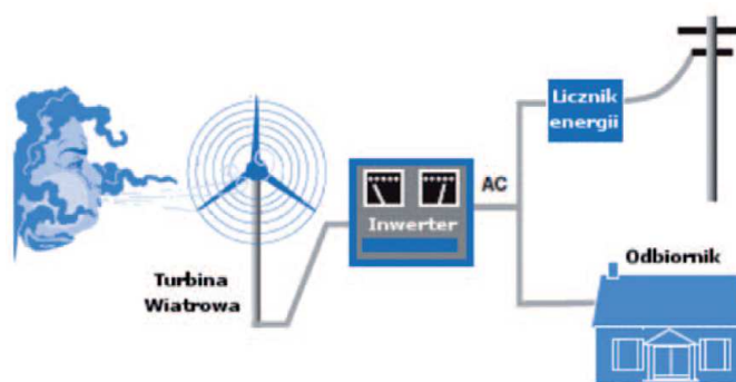
Rysunek 21 System zasilania gospodarstwa domowego zintegrowany z siecią energetyczną 185
