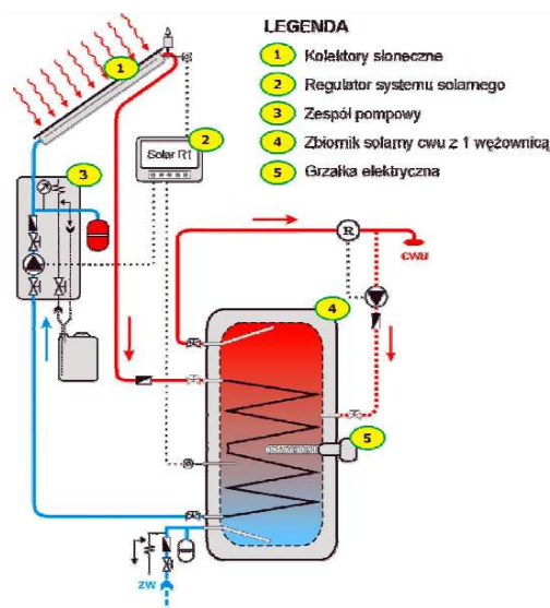
Rysunek 15 Schemat typowej instalacji słonecznej do podgrzewania ciepłej wody użytkowej 174
