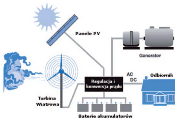
Rysunek 20 Automatyczny (wyspowy) system zasilania gospodarstwa domowego 184
