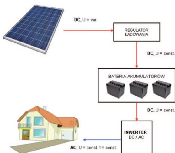
Rysunek 23 Schemat instalacji mieszanej 189 (oznaczenia: DC- prąd stały, AC-prąd przemienny, U- napięcie, f-częstotliwość, var.-zmienne, const.- stałe)
