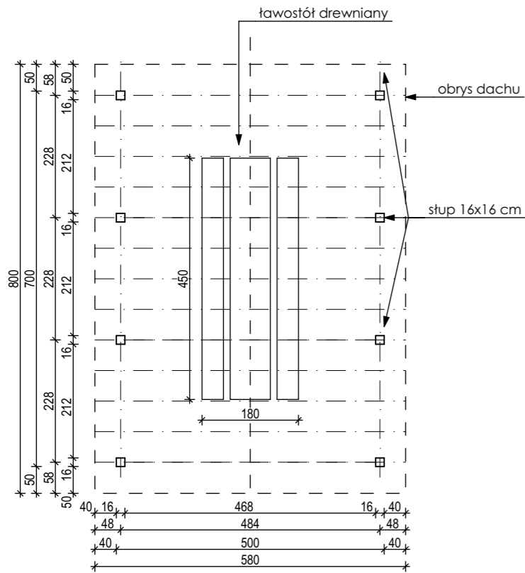
RZUT PRZYZIEMIA
