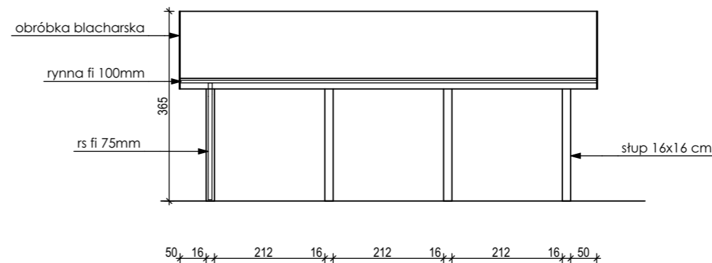
ELEWACJA BOCZNA
