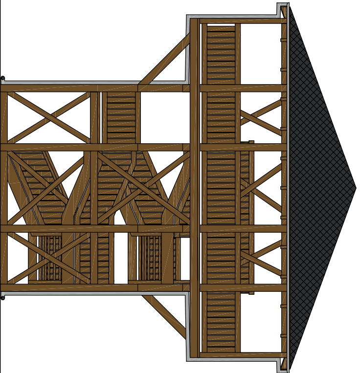
ELEWACJA ZACHODNIA
