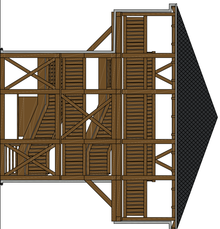
ELEWACJA PÓŁNOCNA
