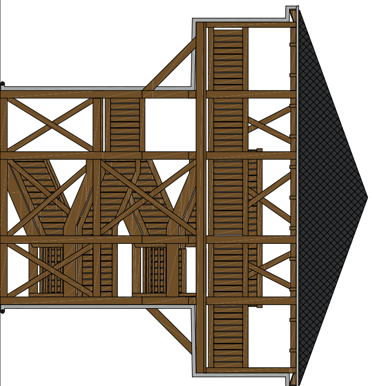
ELEWACJA WSCHODNIA
