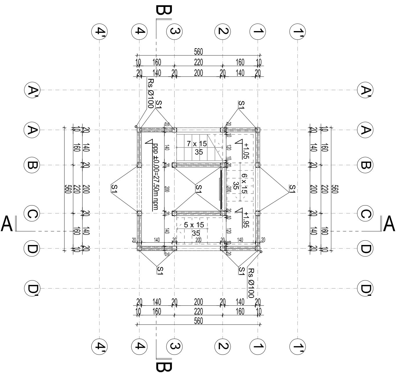
RZUT POZIOMU 0 (PRZYZIEMIENIA)
